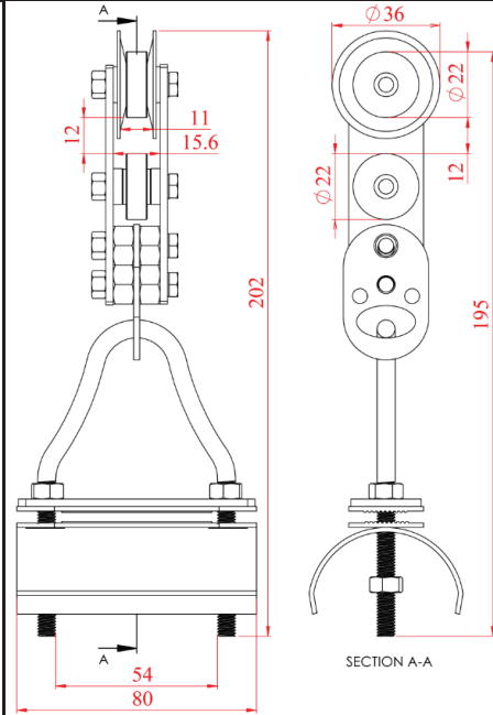
قرقره سیم بکسل با یاتاقان زیر (Wire Rope Steel Trolley for Flat Cable with under Wheel)
