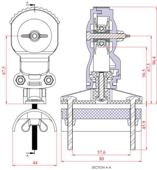
قرقره پلاستیکی سیم بکسل (Wire Rope Plastic Trolley)
